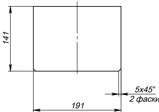
Поз.2 (Ребро)
